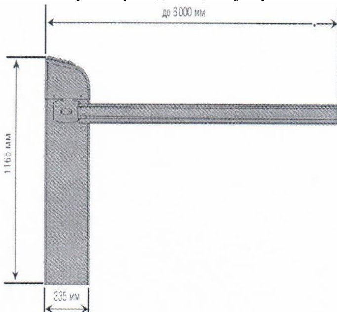
Размеры ограждающего устройства
